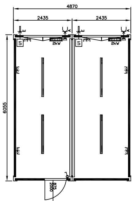
DOPPELANLAGE
