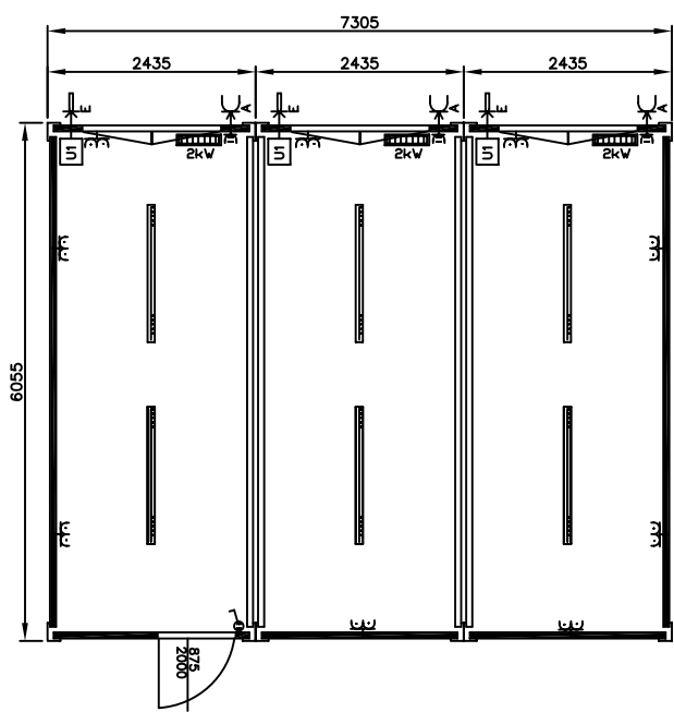
DREIERANLAGE
